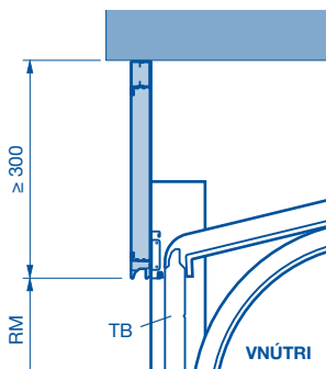
Clona hliníkového rámu
